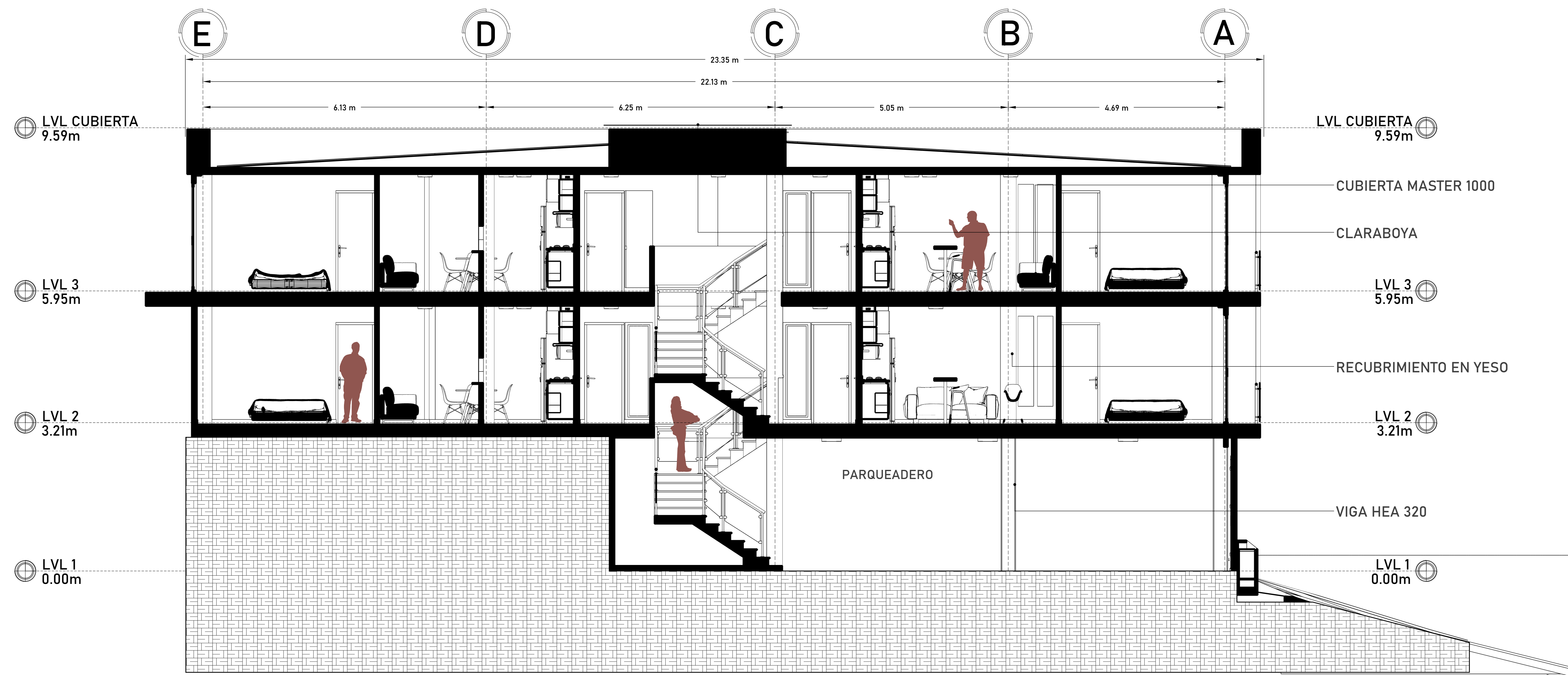
CORTE LONGITUDINAL
