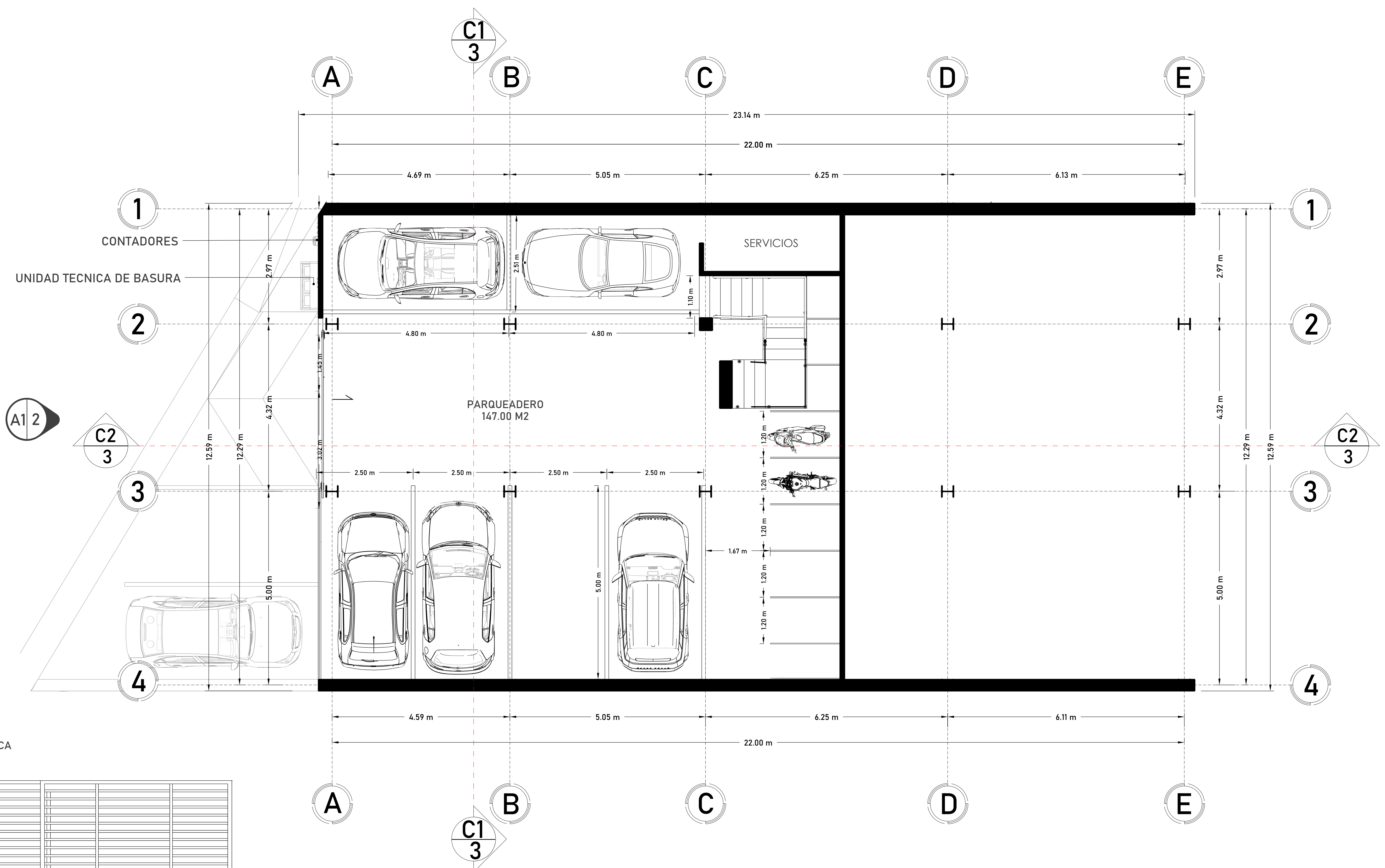
PLANTA ARQUITECTONICA 1 NIVEL
